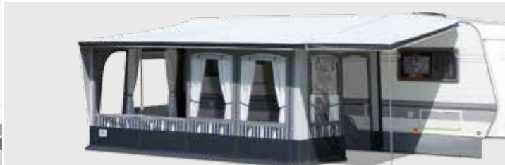
▲ ... Türelement zur Wohnwagenwand versetzt, zwei Elemente der Vorderwand zur Veranda abgeklappt; Tür in eingezogener Seitenwand geöffnet.
